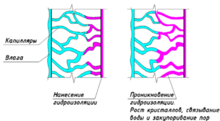
Рис. 1. Проникающая гидроизоляция
