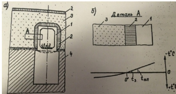
Рис. 1. Схема расположения талых и мерзлых слоев грунта в период, когда прилегающий к секции слой грунта находится на стадии начального промерзания: а) схема расположения талых и мерзлых слоев грунта; б) распределение температуры в грунте насыпи; 1 — стенка звена трубы; 2 — грунт на стадии начального промерзания; 3 — талый грунт насыпи; 4 — талый грунт земляного полотна; t_3 — температура замерзания грунта, t_{кп} — температура начала морозного пучения грунта
