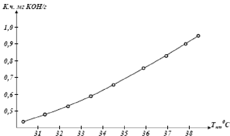
Рис. 2. Соотношение между температурой плавления и кислотным числом саломасов
