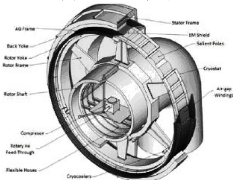
Рис. 1. Проект 10 МВт ветрогенератора на основе MgB_2
