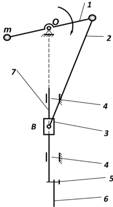
Рис. 1. Схема механизма иглы универсальных и специальных швейных машин где: 1-кривошип; 2-шатун; 3-ползун; 4-подшипник; 5-винт; 6-игла; 7-игловодитель
