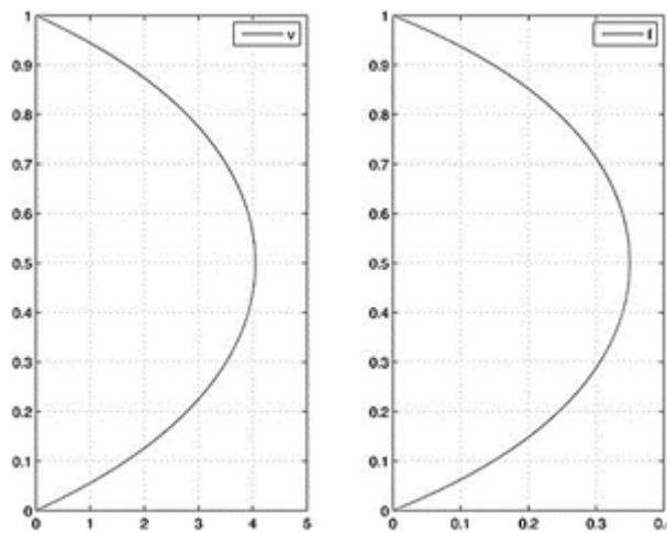
Рис. 2. Re_* = 10^1
