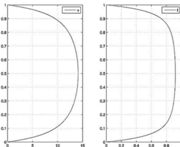
Рис. 3. Re_* = 10^2
