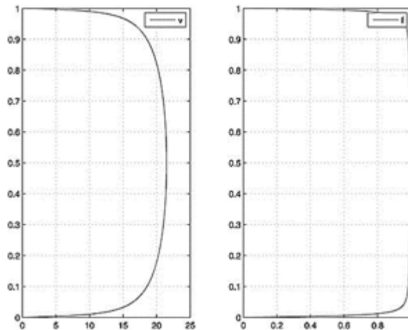
Рис. 4. Re_+ = 10^3
