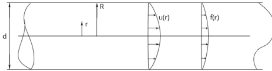
Рис. 1. Модель течения в круглой цилиндрической трубе
