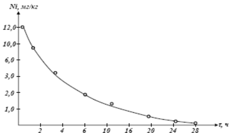
Рис. 1. Влияние продолжительности работы свежего стационарного катализатора № 1 на содержание никеля в саломасе
