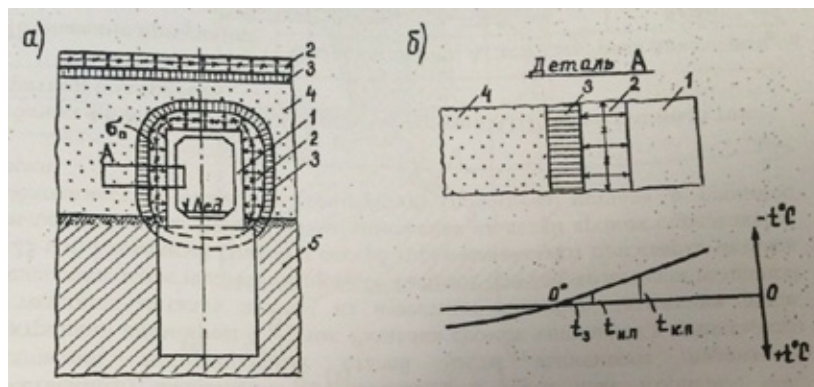
Рис. 2. Схема сил пучения в системе Г-СТ в период, когда прилегающий к секции слой грунта находится на стадии активного промерзания и пучения: а) схемы расположения талых и мерзлых слоев грунта и сил пучения; б) распределение температуры в грунте насыпи; 1 — стенка звена трубы; 2 — грунт на стадии активного промерзания и пучения; 3 — то же начального промерзания; 4 — талый грунт насыпи; 5 — то же грунт земляного полотна; t_{кп} — температура прекращения морозного пучения грунта; t_3 и t_{кп} — обозначения те что и на рис. 1
