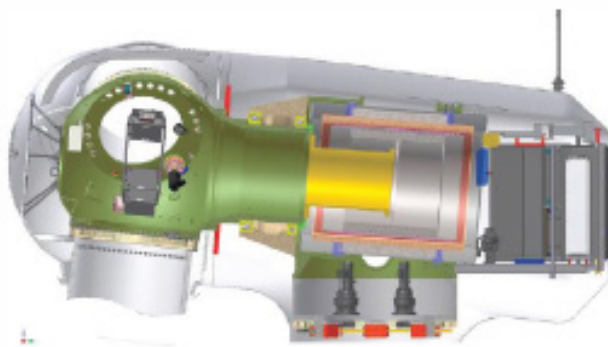
Рис. 4. Внешний вид сверхпроводящего ветрогенератора «Sea Titan»
