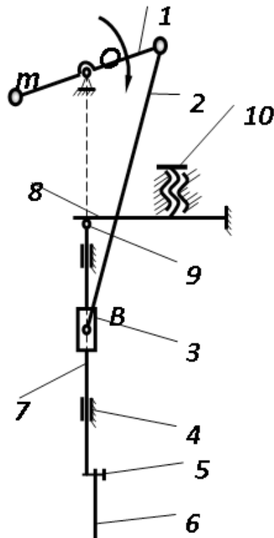
Рис. 2. Механизм иглы с пластичным упругим элементом где: 1-кривошип; 2-шатун; 3-ползун; 4-втулка; 5,10-винт;6-игла; 7-игловодитель; 8-пластинка; 9-шарик
