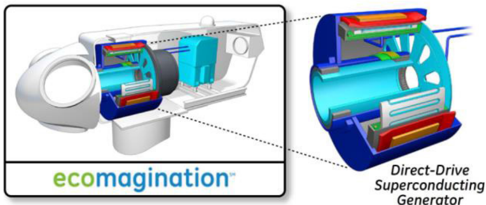
Рис. 3. Схема ветрогенератора мощностью 10 МВт (компания General Electric)
