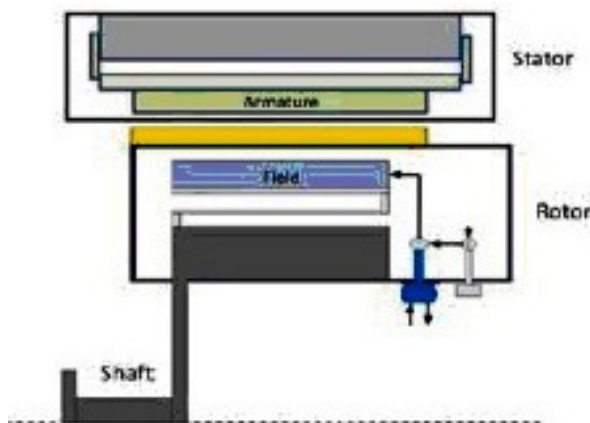
Рис. 5. Схема ветрогенератора мощностью 10 МВт на основе \text{MgB}_2
