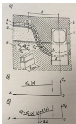
Рис. 3. Схема сил пучения в системе Г-СТ в период, когда прилегающий к секции слой грунта находится на стадии оттаивания. а) схема расположения талых и мерзлых слоев грунта и сил пучения; 1 — секция трубы; 2 — грунт на стадии оттаивания; 3 — то же активного промерзания и пучения; 4 — начального промерзания; 5 — талый грунт насыпи; 6 — тоже земляного полотна. б) вид зависимости \delta_n(X) ; в) то же \delta_\varepsilon(X) .
