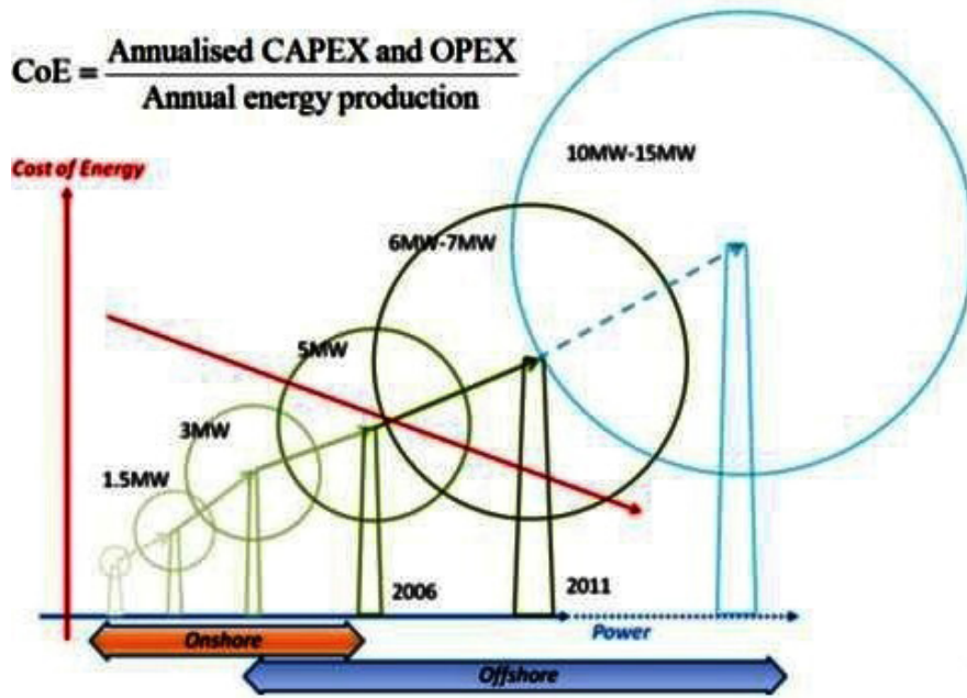
Рис. 2. Эволюция ветрогенераторов
