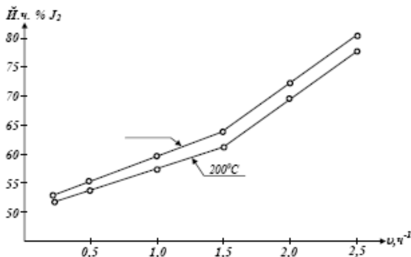
Рис. 3. Зависимость глубины гидрирования от объемной скорости подачи масла
