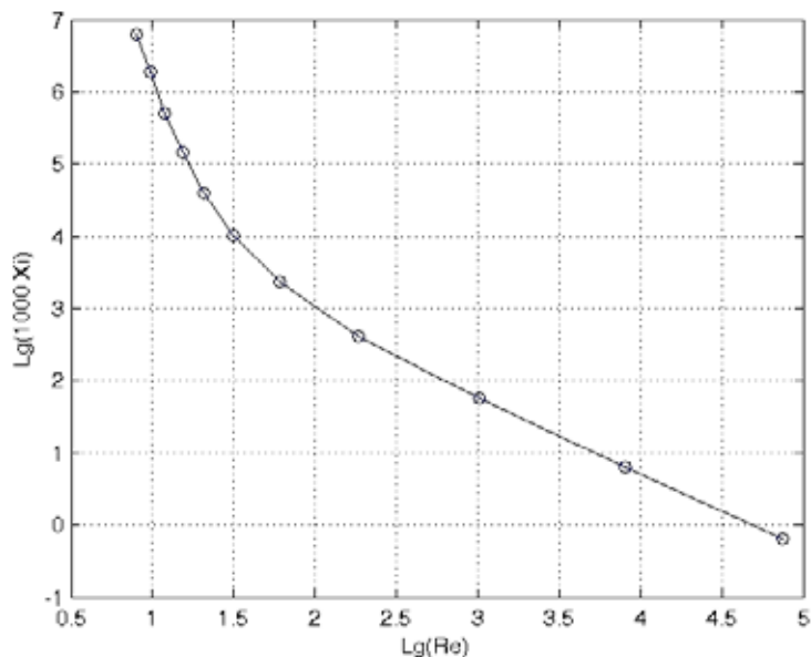
Рис. 6. Коэффициент сопротивления для различных Re
