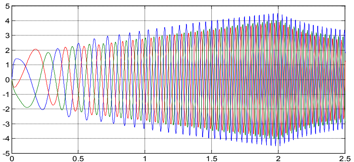
Рис. 17. Токи i_{\alpha}, i_{\beta}, i_{\gamma} на выходе ЛАД
