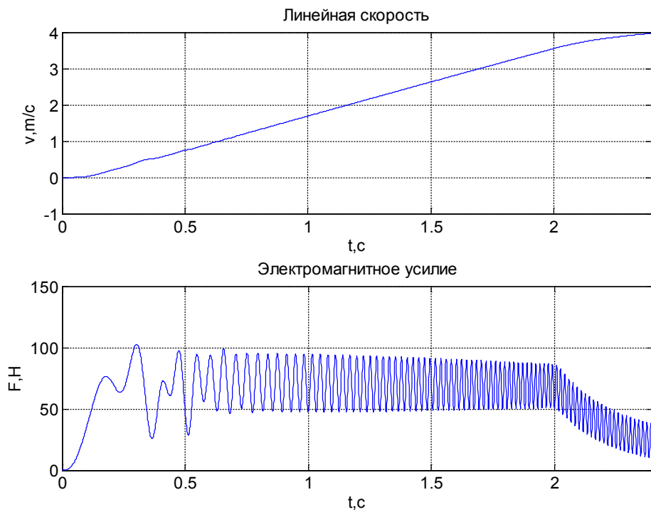
Рис. 20. График скорости и момента в замкнутой системе
