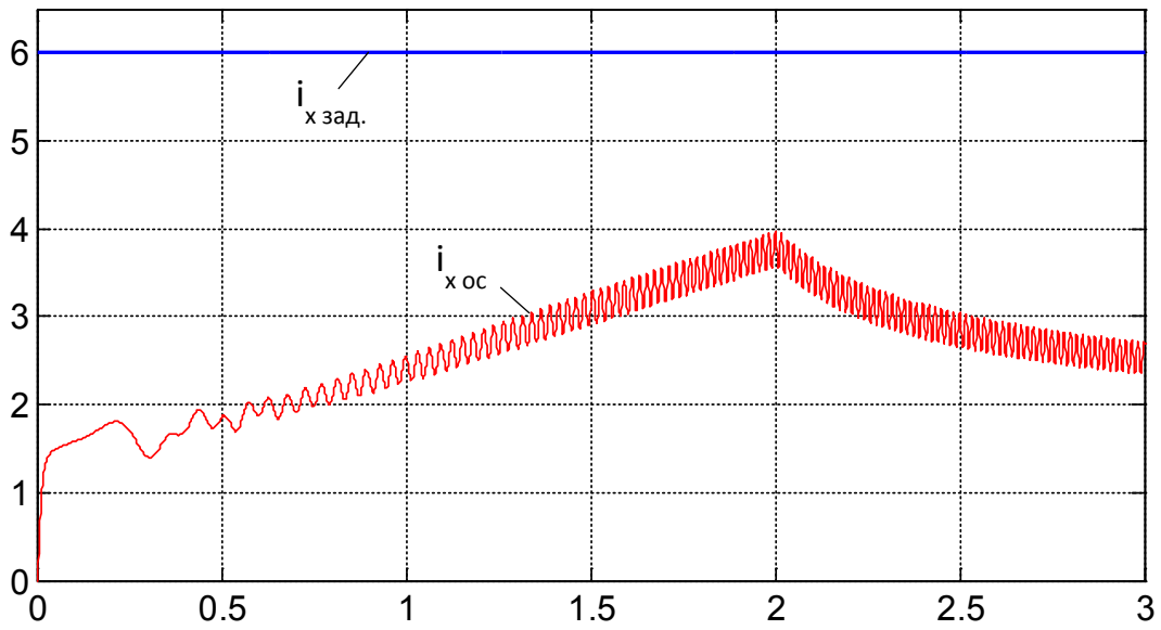
Рис. 12. Токи i_{x \text{ зад.}} и i_{x \text{ ос.}} на входе фильтров ФЭТ и ФОТ
