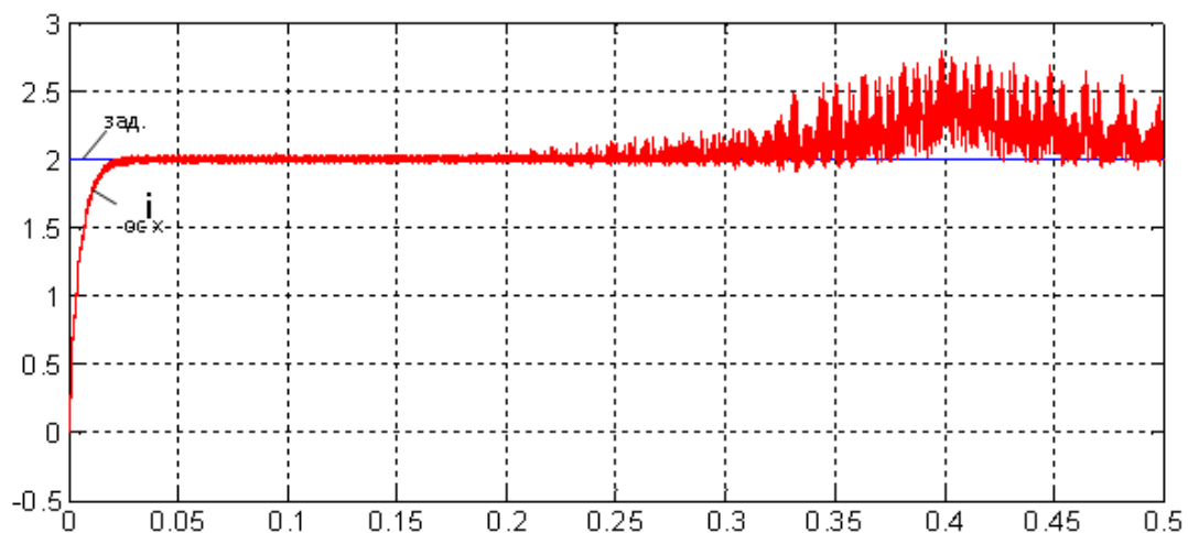
Рис. 12. Токи i_{x\text{зад.}} и i_{x\text{ос}} на входе фильтров ФЗТ и ФОТ
