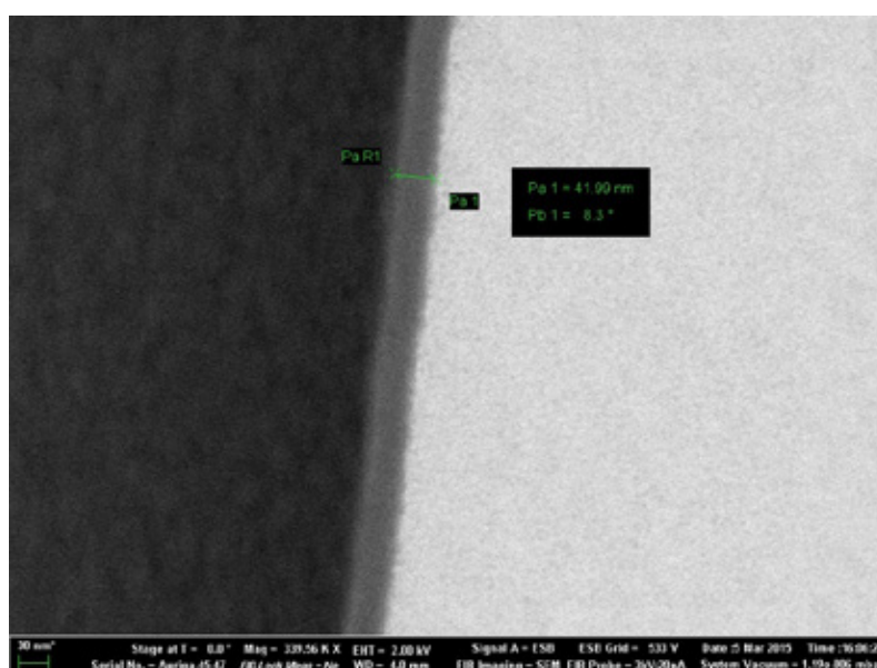
Рис. 5. Электронномикроскопическое изображение пленки оксида алюминия, полученное методом МН на стенке канала МКП
