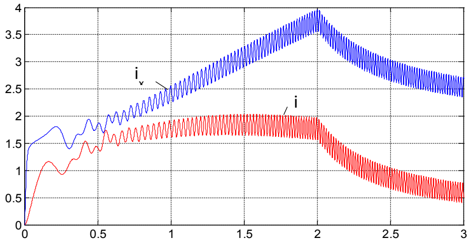
Рис. 19. Токи i_{xoc} , i_{yoc} на выходе прямого преобразователя координат
