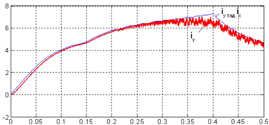
Рис. 13. Токи i_{y\text{зад.}} и i_{y\text{ос}} на входе фильтров ФЗТ и ФОТ
