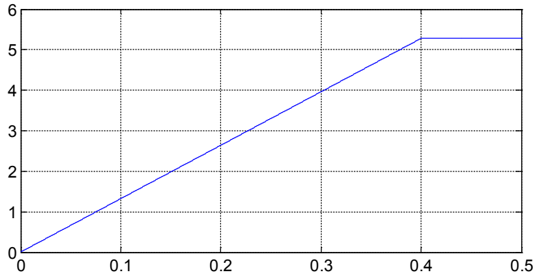
Рис. 2. Сигнал задатчика интенсивности
