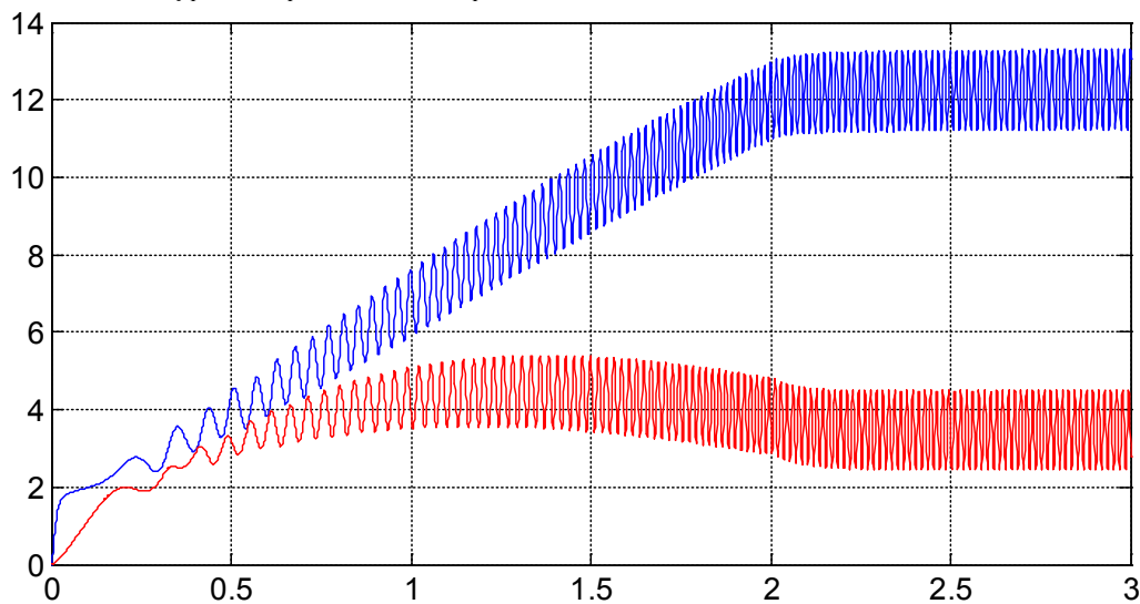
Рис. 10. Токи i_{xoc} , i_{yoc} в разомкнутой системе
