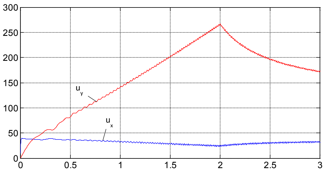
Рис. 14. Напряжения u_x , u_y на выходе регуляторов тока
