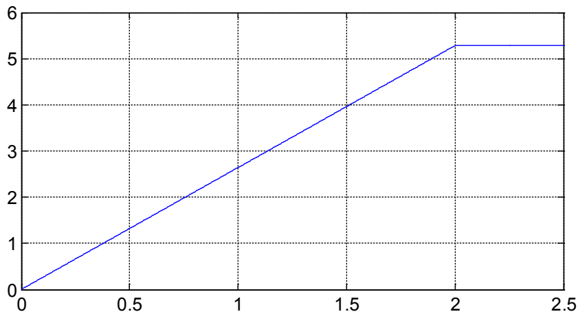
Рис. 2. Сигнал задатчика интенсивности
