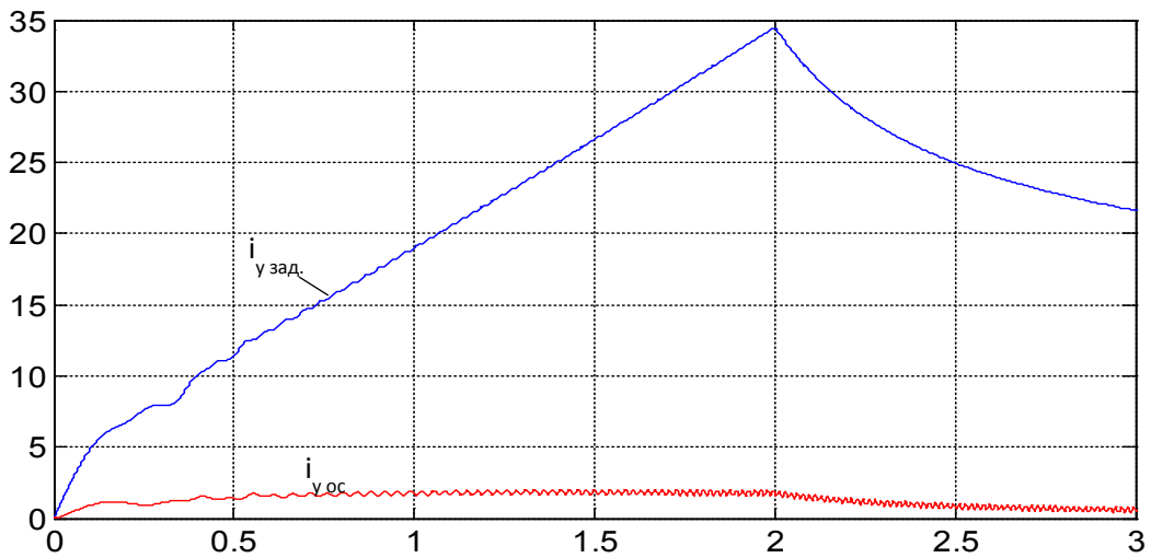
Рис. 13. Токи i_{y \text{ зад.}} и i_{y \text{ ос.}} на входе фильтров ФЭТ и ФОТ
