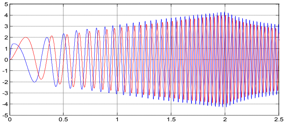
Рис. 18. Токи i_{\alpha} , i_{\beta} на выходе преобразователя ( a, b, c \rightarrow \alpha, \beta )
