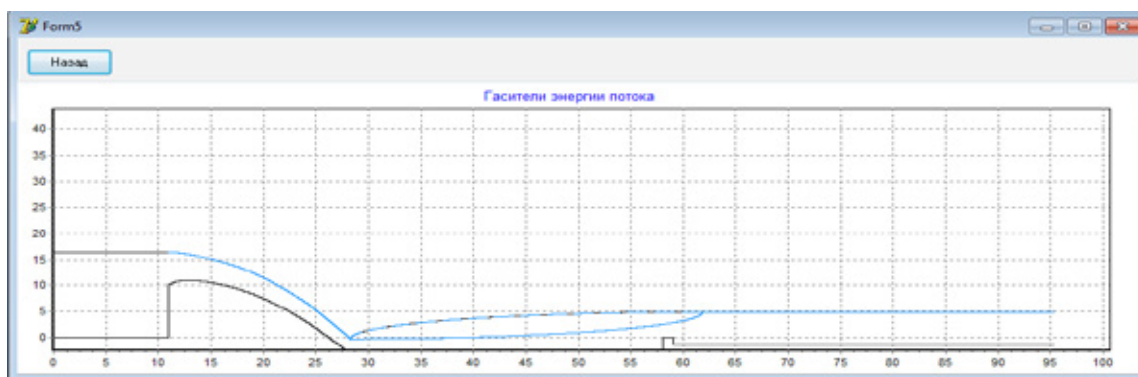
Рис. 6. Расчет и размещение гасителей энергии потока
