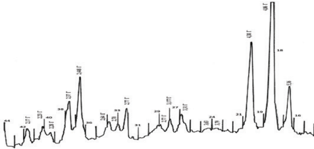
Рис. 1. Рентгенограмма шлама щелочного травления алюминия (в сухом состоянии): Г — гидроаргиллит — Al(OH)_3
