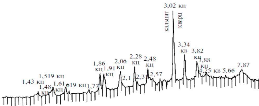
Рис. 3. Рентгенограмма алюмокальциевого шлама: кц — кальцит ( CaCO_3 ); кв — кварц ( SiO_2 )
