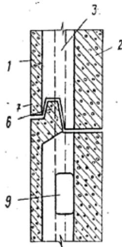
Рис. 2. Горизонтальный стык двух панелей
