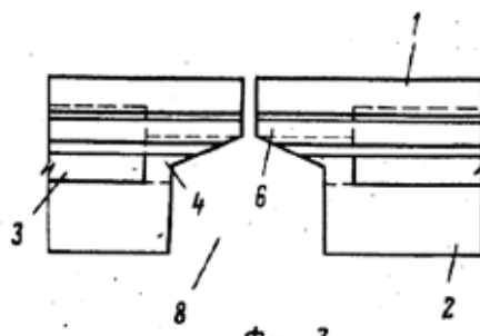
Рис. 3. Вертикальный стык двух панелей. Вид в плане
