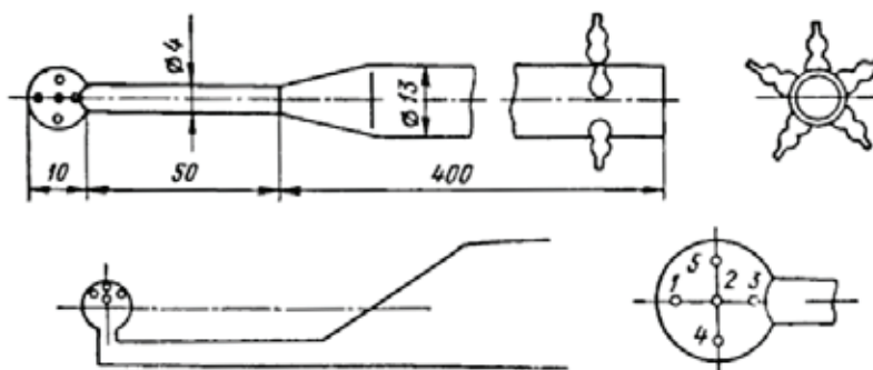
Рис. 2. Типы шаровых зондов
