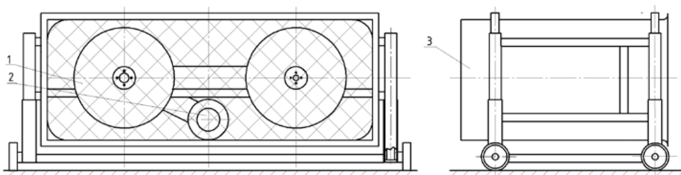
Рис. 3. Схема установки для надува воздуха в подкапотное пространство 1 — Вентилятор; 2 — Электродвигатель; 3-3 — Труба
