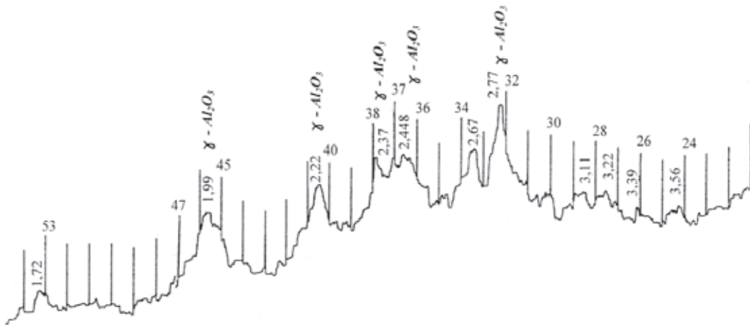
Рис.2. Рентгенограмма шлама щелочного травления алюминия (после термообработки): \gamma-Al_2O_3 — технический глинозем, т. е. Al(OH)_3 \rightarrow \gamma-Al_2O_3 + H_2O \uparrow
