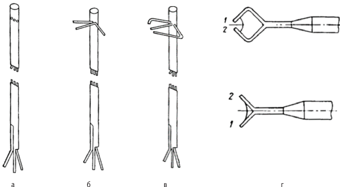
Рис. 1. Насадки для измерения вектора скорости в плоском потоке: а — цилиндрические; б — рожковые; в — хоботковые; г — угломеры
