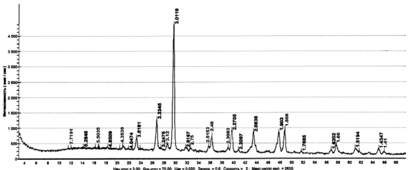
Рис. 4. Рентгенограмма бурового шлама «Покровский горизонт» Интенсивные линии представлены фазами следующих минералов: Кварц, \text{SiO}_2 , d: 3,33; 2,27; 2,21; 1,77; 1,61; 1,52; 1,43 Å, Кальцит, \text{CaCO}_3 , d: 3,82; 3,01; 2,48; 2,27; 2,08; 1,90; 1,52; 1,44 Å.
