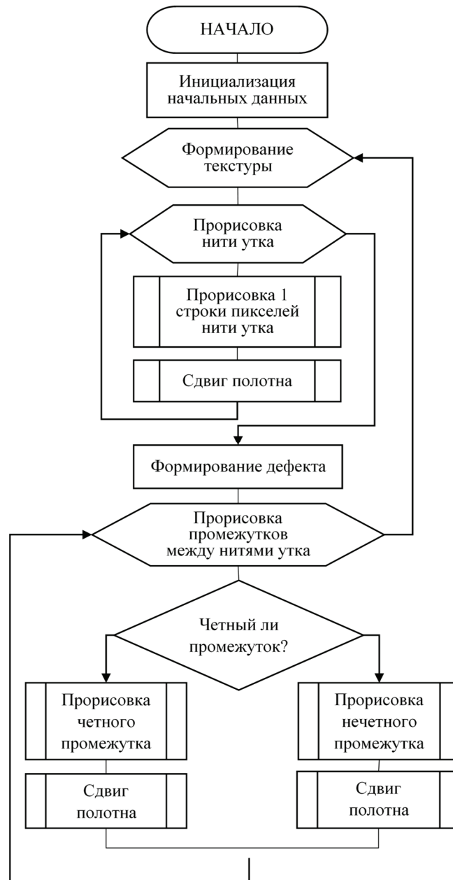
Рис. 3. Блок-схема алгоритма формирования текстуры ткани
