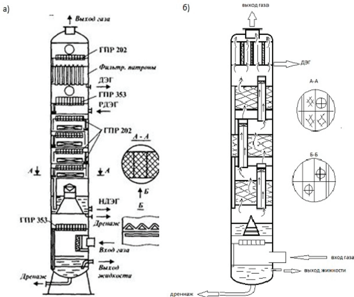
Рис. 1. Принципиальная схема до и после модернизации аппаратов типа ГП-365
