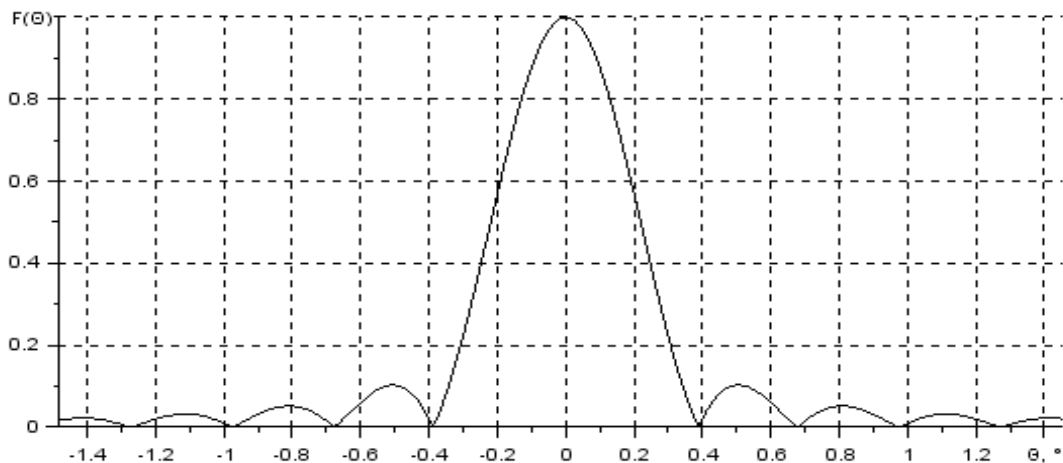
Рис. 4. ДН зеркальной антенны при f_r = 50 ГГц
