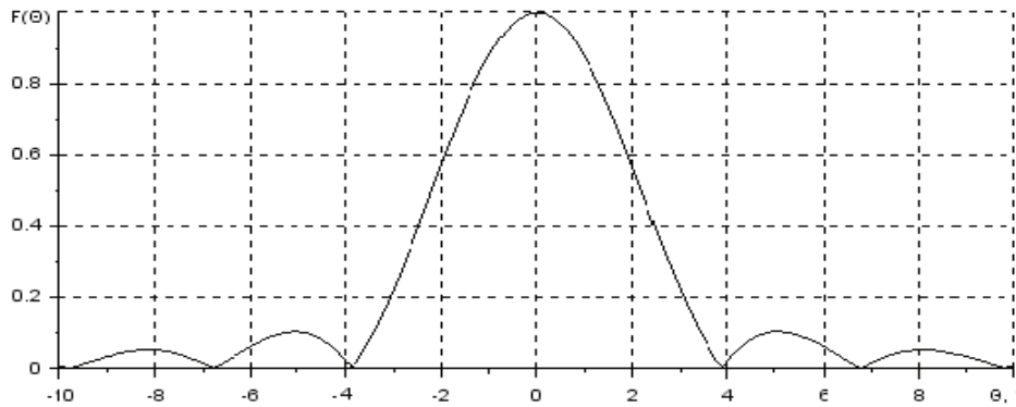
Рис. 3. Нормированная ДН зеркальной антенны
