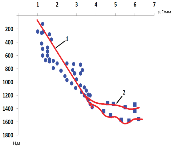
Рис. 5. Изменение удельных электрических сопротивлений в зависимости от глубины в скважинах 154а и 1452а в Балахани, Рамана ■ — глина, ● — дренажные зоны
