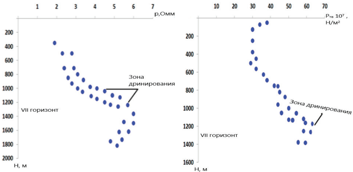
Рис. 6. Изменения удельного электрического сопротивления и твердости глин в скважине Балаханы в зонах дренажа. 1. Продуктивного горизонта VII
