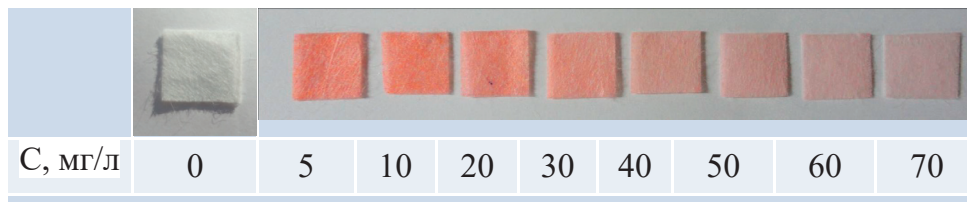
Рис. 2. Цветовая шкала для колориметрического определения нефтепродуктов в воде с красителем судан II
