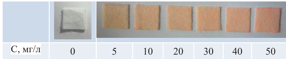
Рис. 1. Цветовая шкала для колориметрического определения нефтепродуктов в воде с красителем судан I
