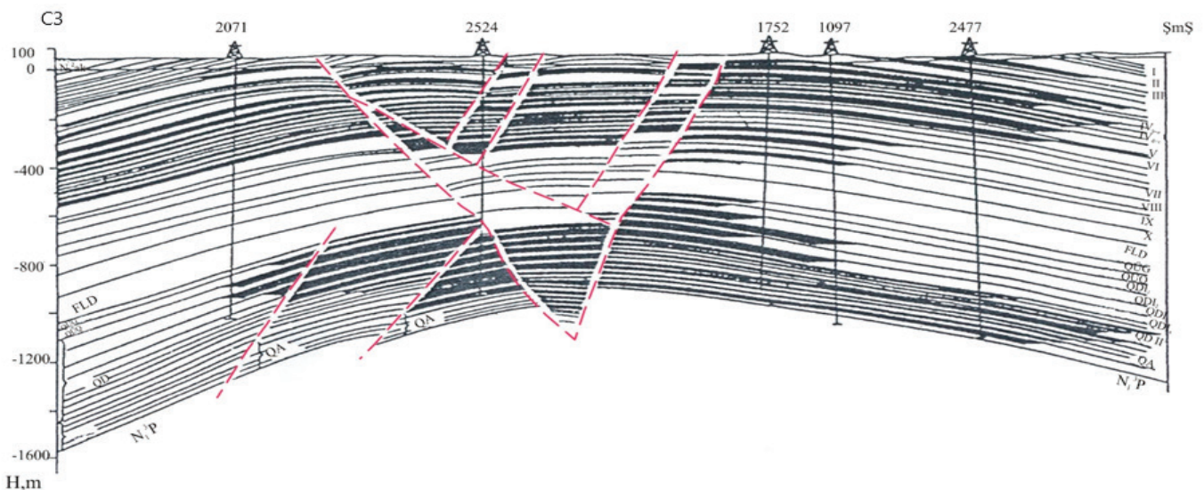
Рис. 3. Поле Балаханы-Сабунчу-Раманы. Геологический профиль по линиям I-I
