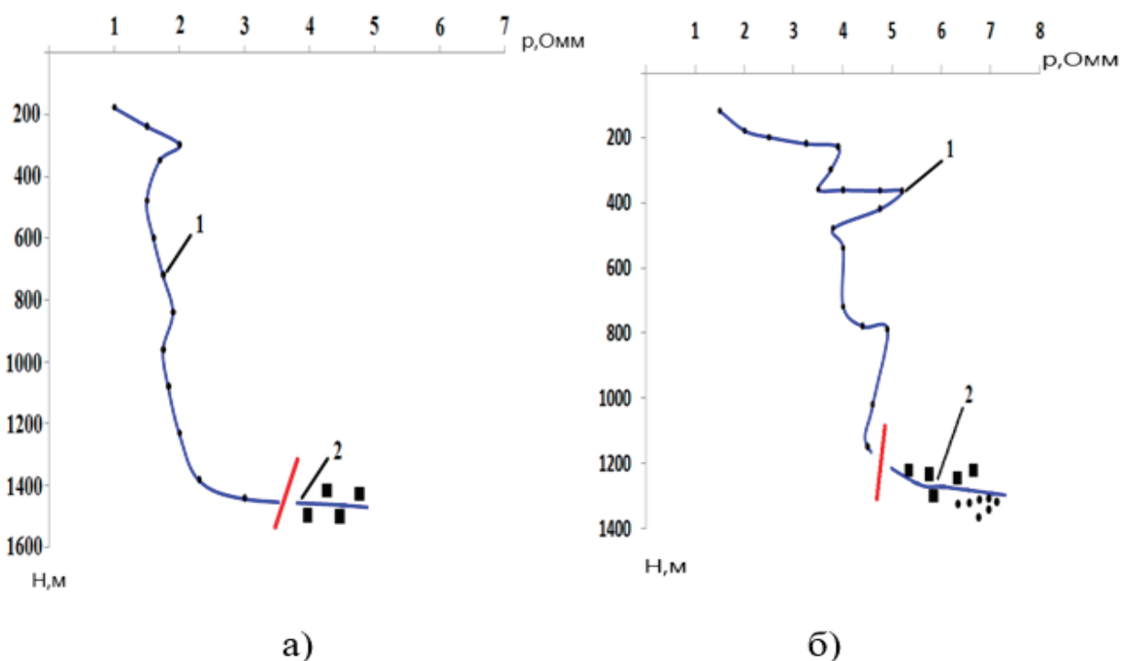
Рис. 4. (а) Изменения удельного электрического сопротивления среднего уровня в Балаханах, (б) Рамана 154а и 1452а.
