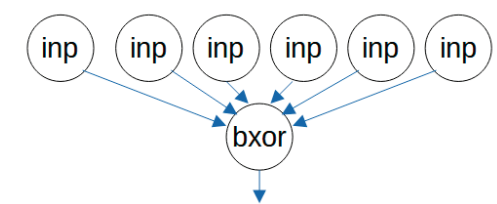
Рис. 3. Нейрон bxor
