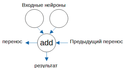
Рис. 4. Нейрон add
