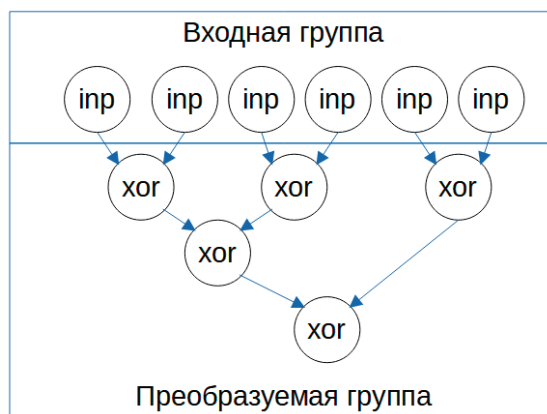
Рис. 2. Обычные нейроны
