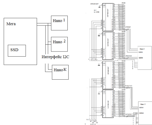
Сурет 3. POV дисплейді басқару схемасы
