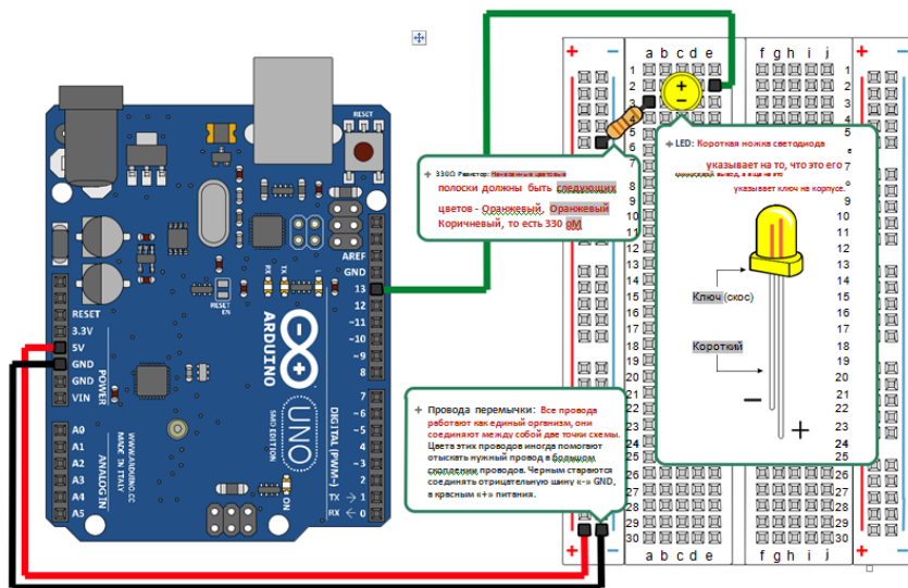
2-расм. Схепада деталларни уланиши
