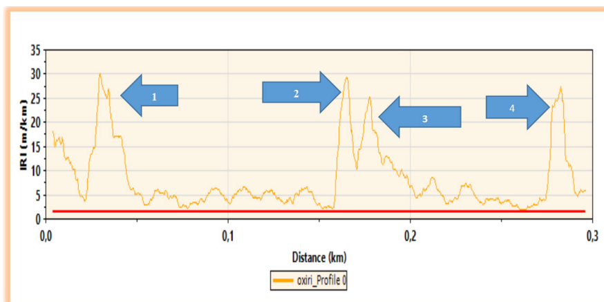
4-расм. Велосипед йўлаги бўйлама профилини нивелир ва рейка ёрдамида ўлчанган диаграммаси
