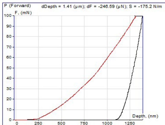
Сур. 1. Электролит құрамына фосфор қышқылын қосу арқылы кальций-фосфат жабыны алынған VT1-0 техникалық титанның индентор көмегімен үлгіге ену тереңдігі мен түсірілген күш арасындағы тәуелділік графигі
