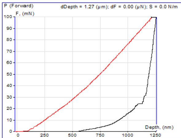
Сур. 3. Электролит құрамына ортофосфор қышқылы мен титан оксидін қосу арқылы кальций-фосфат жабыны алынған BT1-0 техникалық титанның индентор көмегімен үлгіге ену тереңдігі мен түсірілген күш арасындағы тәуелділік графигі
