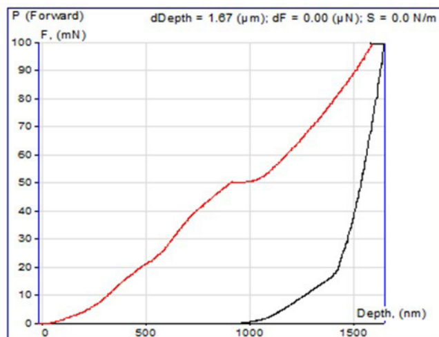
Сур. 2. Электролит құрамына натрий фосфатын қосу арқылы кальций-фосфат жабыны алынған VT1-0 техникалық титанның индентор көмегімен үлгіге ену тереңдігі мен түсірілген күш арасындағы тәуелділік графигі
