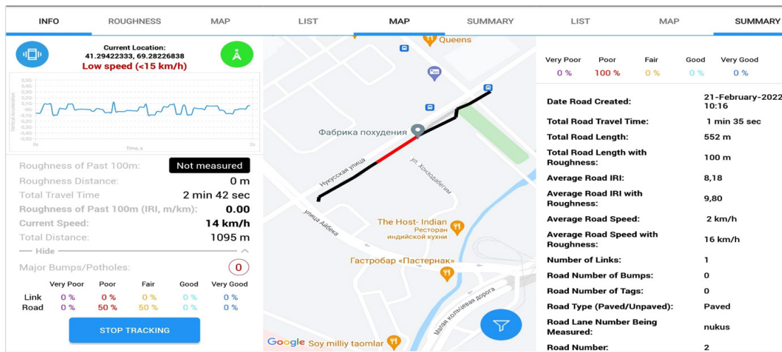
7-расм. Велосипедда йўл раванлигини аниқлаш жараёни
