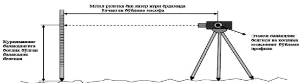
1-Расм. Қоплама юзасининг бўйлама профилини нивелир ва рейка ёрдамида ўлчаш
