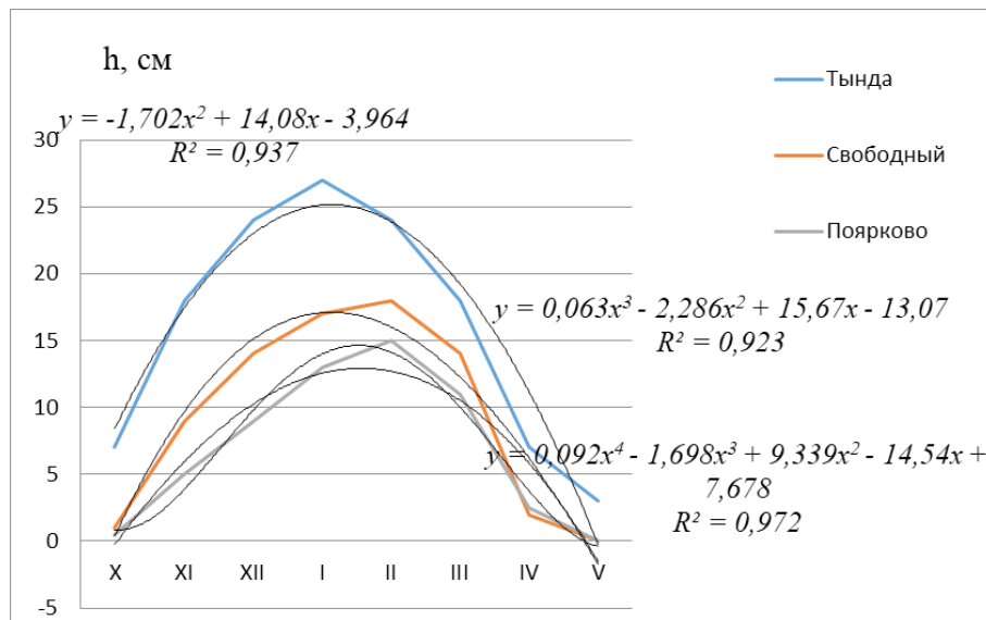
Рис. 4. Высота снежного покрова
