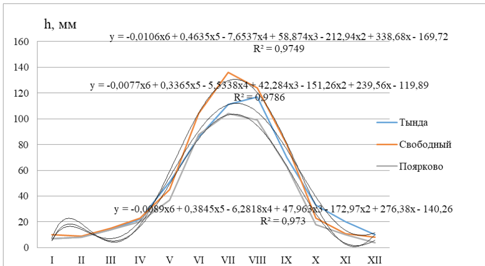
Рис. 2. Распределение осадков по месяцам
