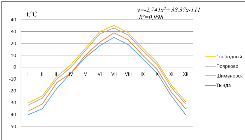
Рис. 1. Изменение температуры воздуха (°C) по месяцам года
