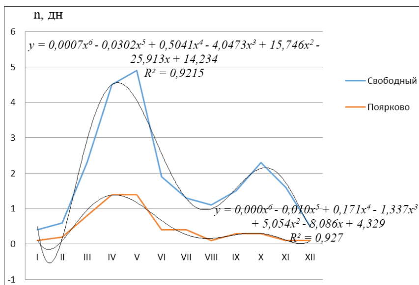
Рис. 3. Число дней с сильным ветром, ( V > 15 м/с)
