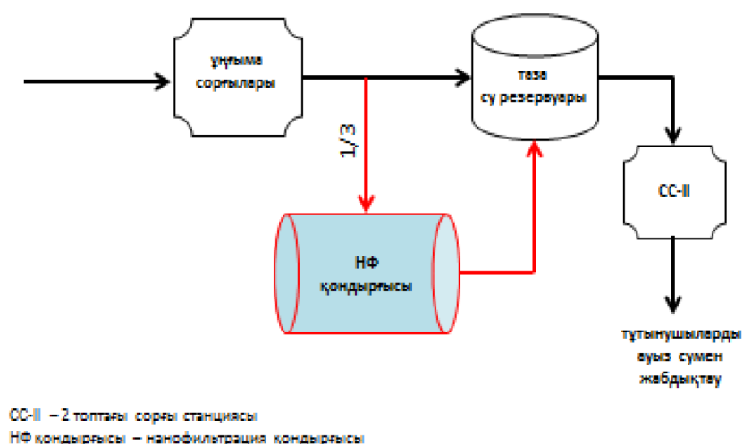
Сурет 2. Ауыз суды тазарту технологиясының схемасын жетілдіруге арналған ұсыныстар
