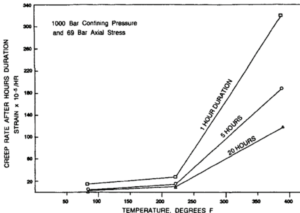
Рис. 1 Влияние температуры на ползучесть соли [9]
