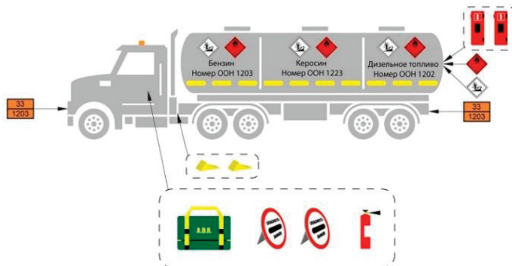
Рис. 12. Оборудование автомобиля для перевозки ОГ
