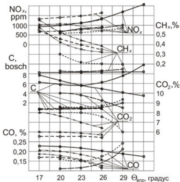
Рис. 1. Влияние применения КПГ и РОГ, МТЭ и ЭТЭ на содержание токсичных компонентов в ОГ дизеля 4Ч 11,0/12,5 зависимости от изменения установочного угла опережения впрыскивания топлива при n = 2200 \text{ мин}^{-1} ; ■ — дизельный процесс; ○ — газодизельный процесс; × — газодизельный с РОГ 10%; △ — газодизельный с РОГ 20%; ○ — ЭТЭ; ○ — МТЭ
