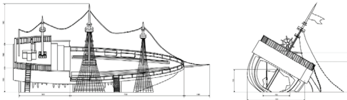
Рис. 3. Размеры корабля
