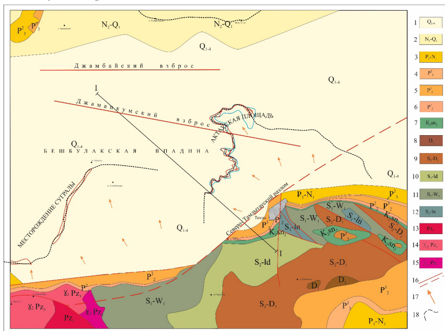
Рис. 1. Геологическая карта северного обрамления гор Тамдытау: 1 — Четвертичные отложения. Золотые барханные пески, суглинки и пролювиальные конгломераты; 2 — Плиоцен — нижний отдел четвертичной системы нерасчлененные пески, конгломераты, глины; 3 — Олигоцен-миоцен нерасчлененные. Красноцветные алевролиты и алевроплиты; 4 — Средний олигоцен. Красные глины и песчаники; 5 — Верхний эоцен. Зеленовато серые глины, редко песчаники; 6 — Средний эоцен. Мергели, мергелистые глины; 7 — Верхний сенон. Пески, песчаники, ракушники; 8 — Нижний девон. Известняки, доломиты; 9 — Верхний силур-нижний девон нерасчлененные. Известняки, песчаники; 10 — Верхний силур-нижний девон нерасчлененные. Лудловский ярус. Конгломераты, гравелиты, песчаники,
