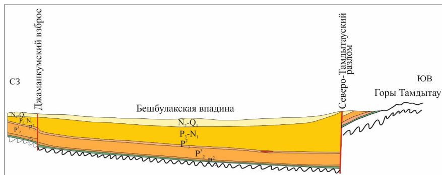
Рис. 2. Геологический разрез по линии I-I
