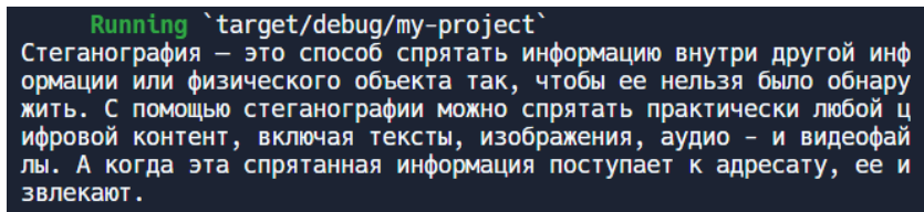
Рис. 4. Декодированная информация
